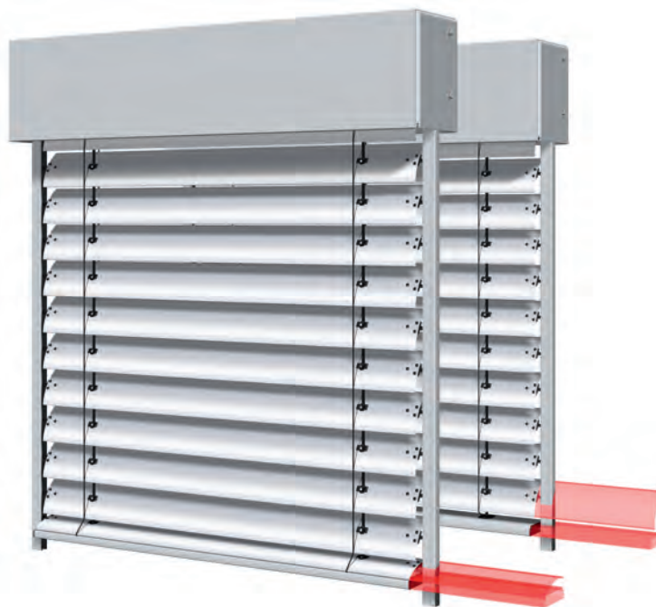
Bild 10: Teilungsausgleich
