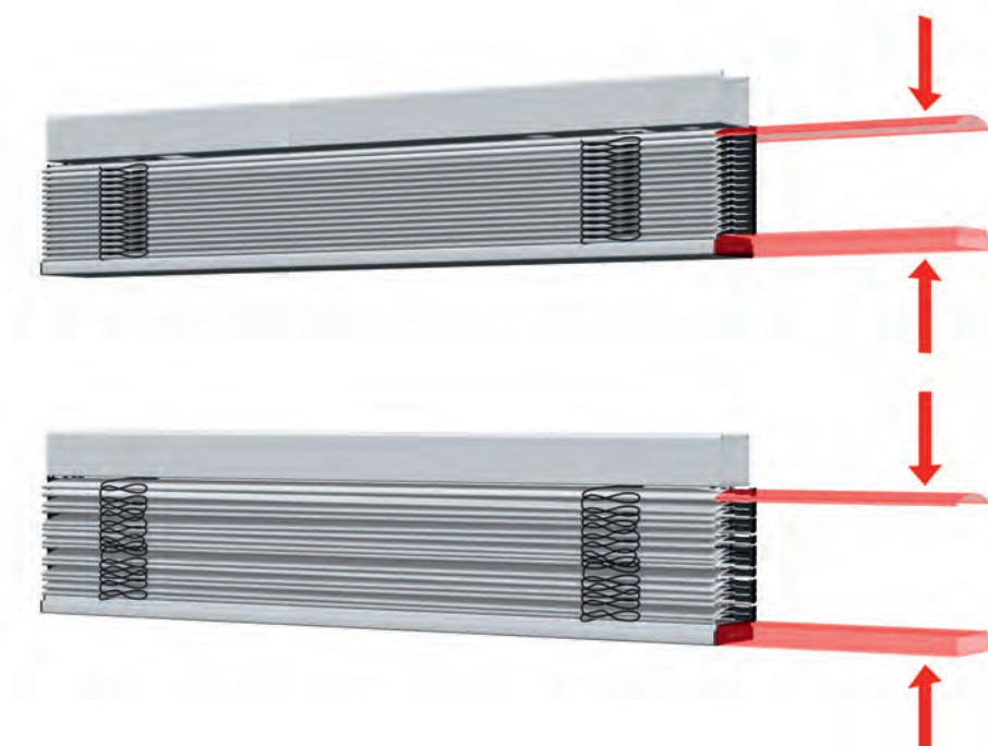
Bild 8: Unterschiedliche Lamellenpakethöhen durch erhöhten Paketaufbau (Unterschiene gerade)
