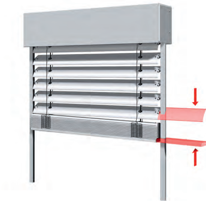
Bild 7: Schräglauf der Unterschiene (bei parallelem Lamellenpaket)
