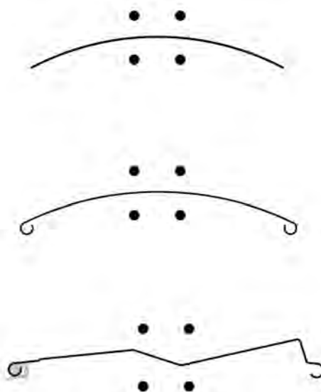
Bild 3: Sichtflächendefinition gängiger Raffstorelamellen (Beschichtungen von Stanzungen, Längsschnitten und Kanten sind nicht Stand der Technik). Zu beachten: Durch unterschiedliche Chargen können die Farben unterschiedlich wirken – was insbesondere bei profilierten Lamellen zu unterschiedlichen Farbwahrnehmungen führen kann.
