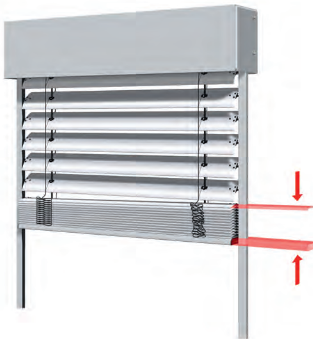
Bild 9: Paketparallelität (Lamellenpaket schief, Unterschiene gerade)
